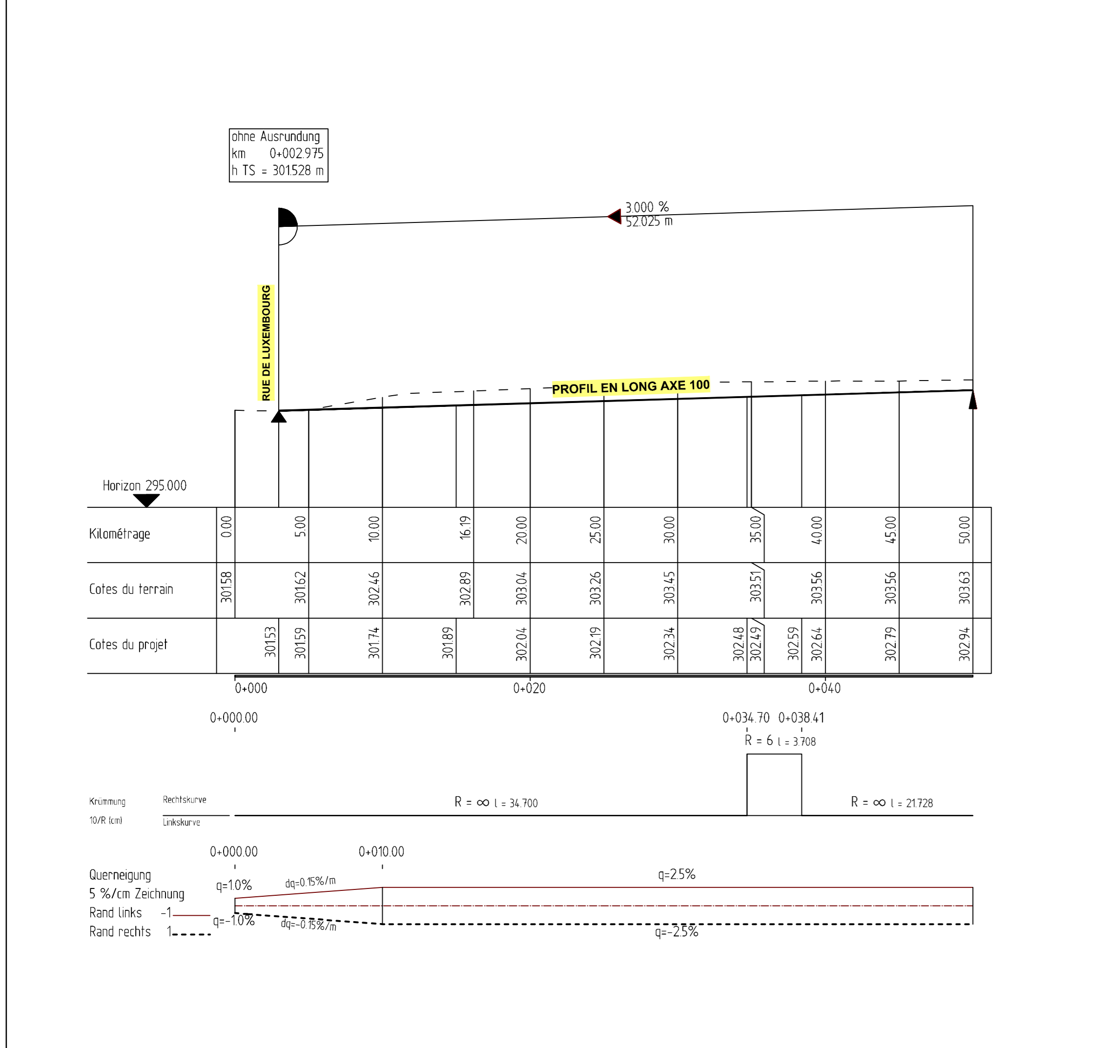
PROFIL EN LONG - AXE 100 - STAT 0+000 - 0+050, 1:250/250
