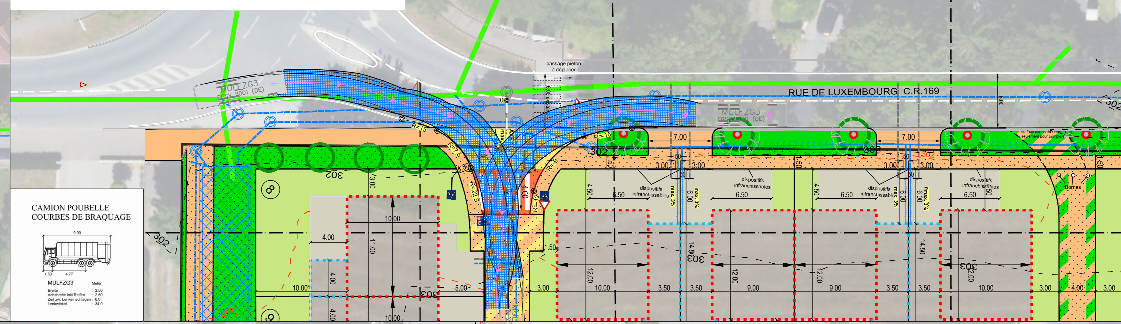
PLAN SITUATION - COURBE DE BRAQUAGE, 1:250
